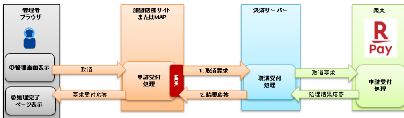
図 3-2-5 MDK 利用時システム処理概要図（楽天ペイ（オンライン決済）V2 取消要求）
