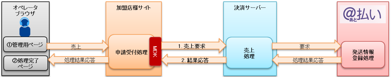
図 3-2-2 MDK 利用時システム処理概要図 (売上)
