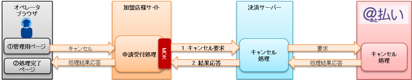
図 3-2-3 MDK 利用時システム処理概要図 (取消)
